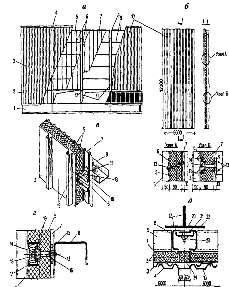
Рис. 6.37. Стена из панелей укрупнительной сборки: а — фасад; б — стеновая панель, ее характерные узлы; в — крепление внутренней обшивки и утеплителя к раме панели; г — вертикальный разрез панели и детали крепления; д — крепление панелей к колоннам каркаса и заделка вертикального стыка; 1 — цокольная панель; 2 — элемент угловой окантовки; 3 — наружная обшивка; 4 — кашельник; 5 — два слоя плит из пенополистирола (1 × 1,8 м); 6 — обрешетка от смещения плит утеплителя; 7 — внутренняя обшивка; 8 — стойки несущей рамы; 9 — ригели несущей рамы; 10 — стеновая панель; 11 — колонна каркаса; 12 — опорный столик, приваренный к колонне; 13 — самонарезающие болты; 14 — болт М10; 15 — пластинка, приваренная к болту; 16 — трубчатая втулка; 17 — прижимные накладки; 18 — утепление минеральной ватой; 19 — шайбы; 20 — пластина с болтами М6; 21 — затягиваемая пластина; 22 — зажимная скоба; 23 — гайка М16; 24 — брусок из пенополистирола
