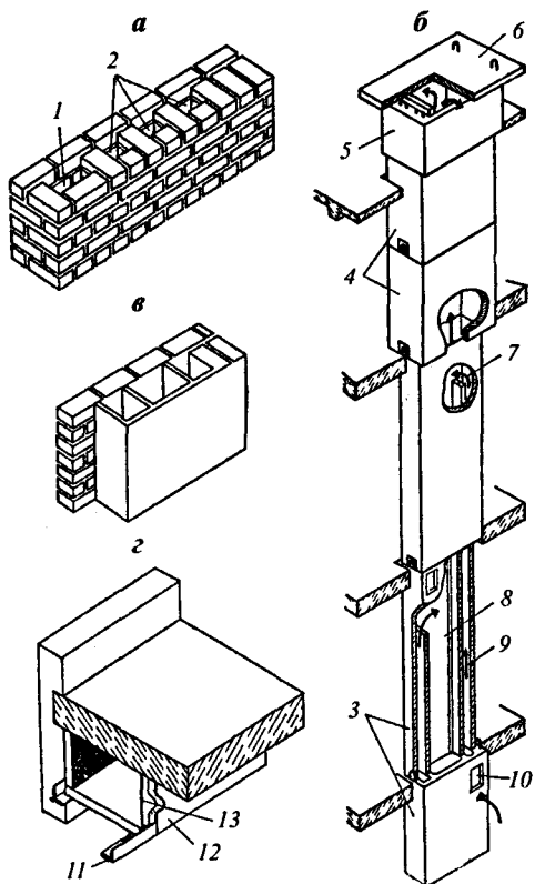
Рис. 4.17. Вентиляционные каналы:
