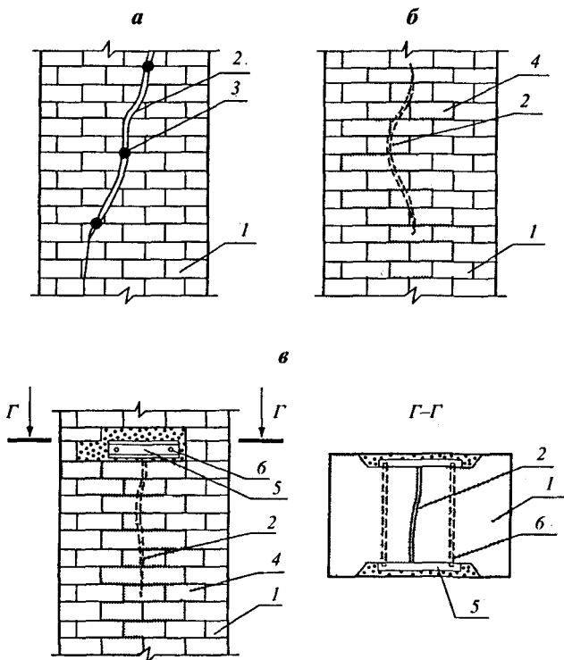
Рис. 9.2. Заделка трещин в кирпичных стенах: а — инъецированием цементным раствором трещин (с раскрытием до 10 мм); б — вставкой простых кирпичных «замков»; в — вставкой кирпичных «замков» с металлическими «якорями»; 1 — усиливаемый участок стены; 2 — трещина; 3 — отверстия диаметром 30 мм и глубиной 100 мм для установки инъекторов; 4 — кирпичный «замок» толщиной \frac{1}{2} кирпича, устанавливаемый с обеих сторон стены; 5 — «якорь» из прокатного профиля; 6 — стяжные болты
