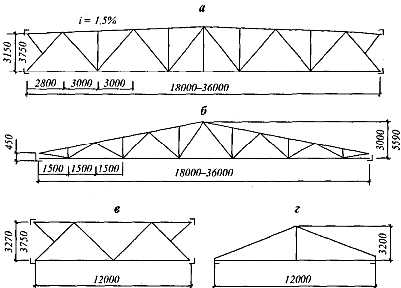
Рис. 6.25. Схемы стальных стропильных и подстропильных ферм: a — с параллельными поясами для плоских покрытий; б — треугольная для неутепленных покрытий; в — подстропильная с параллельными поясами; г — подстропильная треугольная
