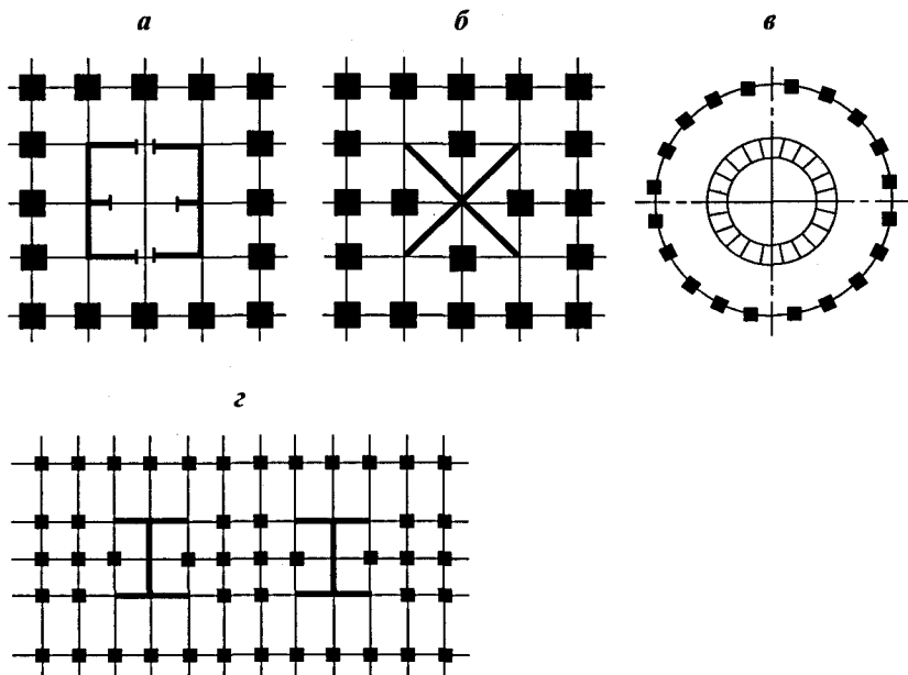
Рис. 4.9. Схема зданий со связевыми элементами: а — коробчатыми; б — X-образными; в — круглыми; г — двутавровыми
