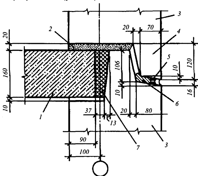
Рис. 4.4. Конструкция горизонтального стыка однослойных стеновых панелей: 1 — железобетонная панель перекрытия; 2 — цементный раствор; 3 — стеновая панель; 4 — противодождевой барьер; 5 — герметизирующая мастика (тиоколовая или полиизобутиленовая УМС-50); 6 — поризол или гернит; 7 — термовкладыш в гидроизоляционной оболочке
