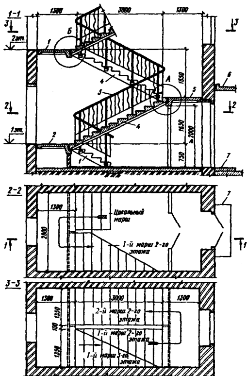
Рис. 3.56. Двухмаршевая лестница (разрез и поэтажные планы):
