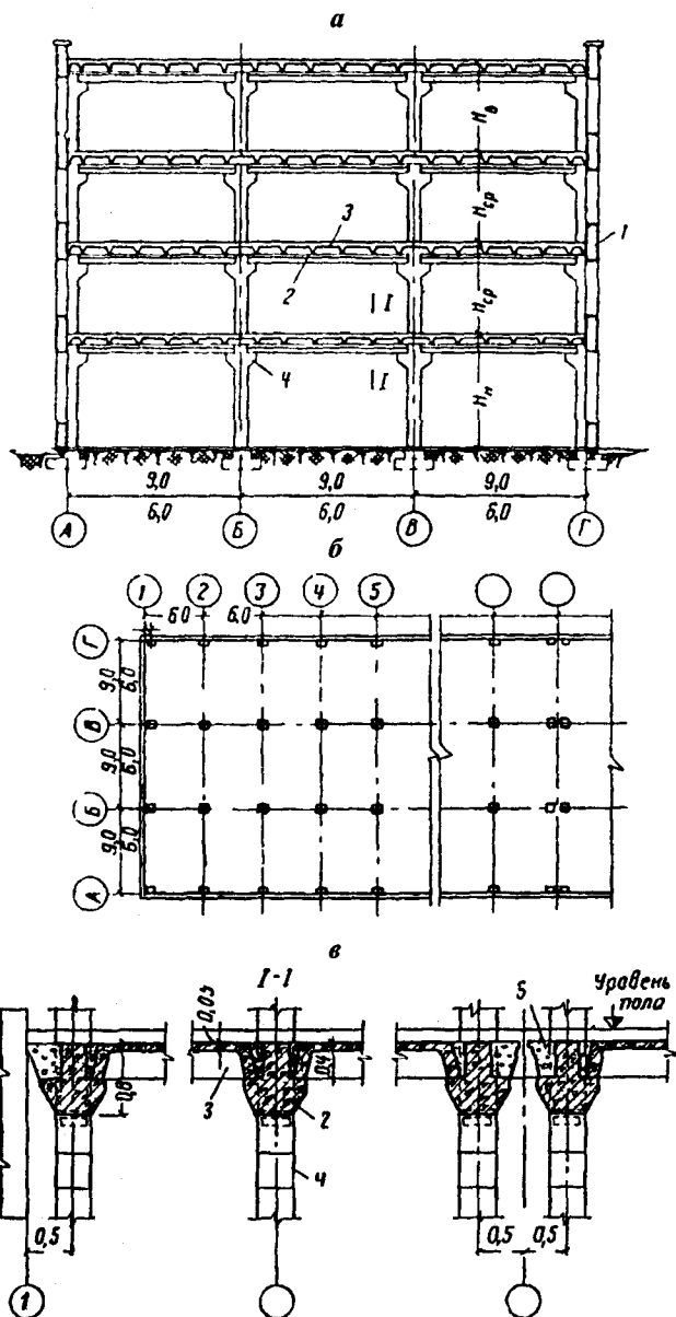
Рис. 6.18. Многоэтажное здание с балочными перекрытиями: а — поперечный разрез здания с плитами, опёртыми на полки ригелей; б — план; в — детали каркаса; 1 — самонесущая стена; 2 — ригель с полками; 3 — ребристые плиты; 4 — консоль колонны; 5 — железобетонный элемент для заполнения деформационных швов
