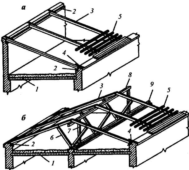
Рис. 3.49. Крыши из наслонных стропил: 1 — чердачное перекрытие; 2 — мауэрлат; 3 — стропильная нога; 4 — кобылка, 5 — обрешетка; 6 — подкос; 7 — стойка; 8 — прогон; 9 — лежень
