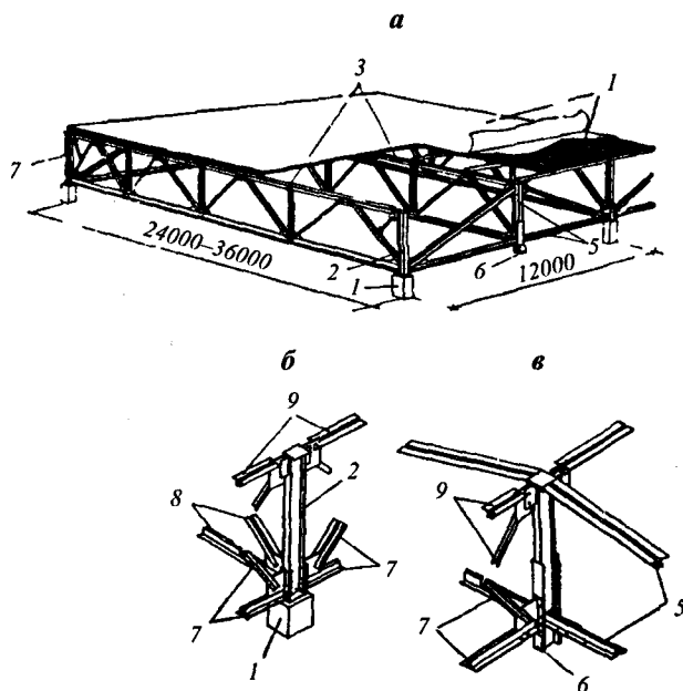
Рис. 6.30. Сопряжение стальных стропильных и подстропильных ферм: а — схема установки ферм; б — сопряжение ферм на оголовке колонн; в — сопряжение ферм в пролете; 1 — колонна; 2 — надопорная стойка; 3 — стропильные фермы; 4 — покрытие; 5 — подстропильная ферма; 6 — столик для опирания стропильной фермы; 7 — нижний узел стропильной фермы; 8 — нижний узел подстропильной фермы; 9 — верхние узлы стропильных ферм
