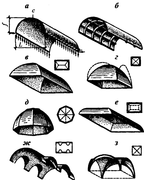
Рис. 3.62. Основные формы сводов:
