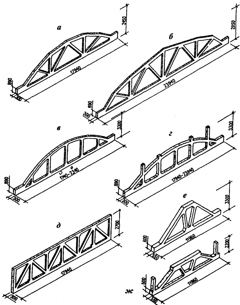
Рис. 6.14. Железобетонные фермы:
