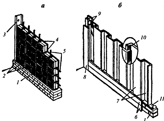
Рис. 3.38. Перегородки: а — из стеклоблоков; б — из профильного стекла; 1 — кирпичный цоколь; 2 — стеклоблоки; 3 — стальная обвязка, закрепленная дюбелями; 4 — швы для раствора; 5 — арматура; 6 — деревянная обшивка; 7 — профильное стекло швеллерного сечения; 8 — наличник; 9 — бруски обвязки; 10 — клеящая пленка; 11 — резиновая прокладка
