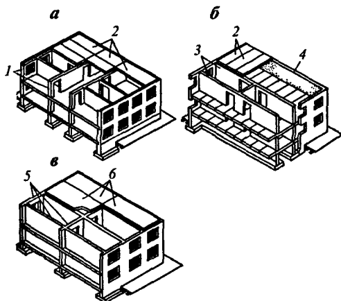
Рис. 3.3. Бескаркасная система зданий: а — с продольным расположением несущих стен; б — с поперечным расположением несущих стен; в — перекрестная; 1 — наружные и внутренние несущие стены; 2 — плиты междуэтажных перекрытий; 3 — наружные самонесущие стены; 4 — торцовая несущая стена; 5 — продольные и поперечные несущие стены; 6 — плиты перекрытия, опертые по контуру
