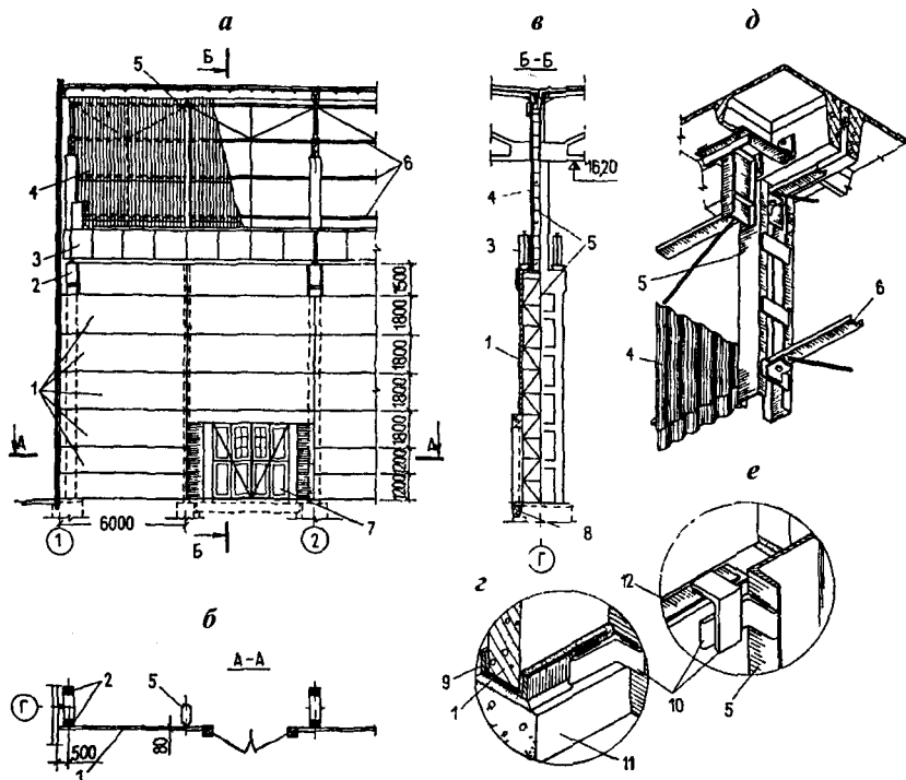
Рис. 6.50. Крупнопанельные перегородки:
