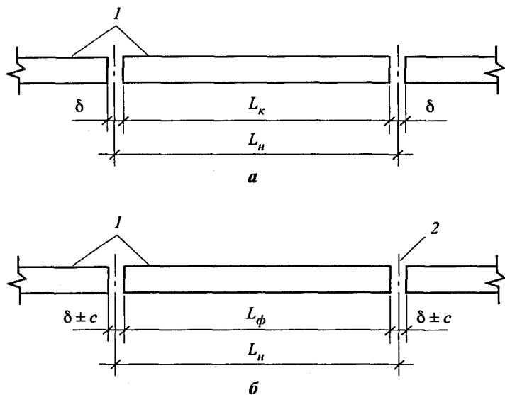
Рис. 1.2. Размеры конструктивных элементов: а — номинальный и конструктивный; б — натурный; 1 — конструктивные элементы; 2 — зазор
