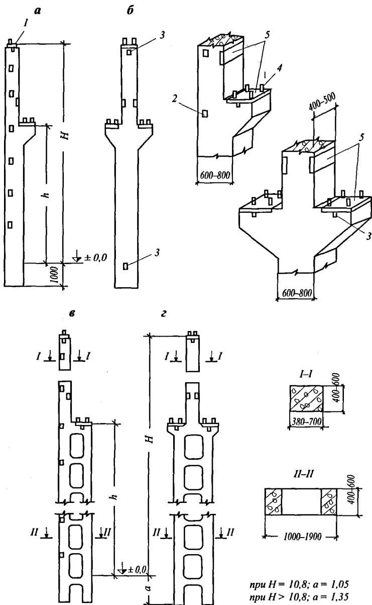
Рис. 6.10. Сборные железобетонные колонны для крановых пролетов: а, б — одноветвевые (крайние и средние); в, г — двухветвевые; 1 — закладные детали для крепления балок или ферм покрытия; 2 — то же для приварки анкеров, скрепляющих стену с колоннами; 3 — риски; 4 — анкерные болты; 5 — закладные детали для крепления подкрановых балок
