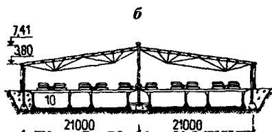
Рис. 7.1. Коровник на 600 голов:
