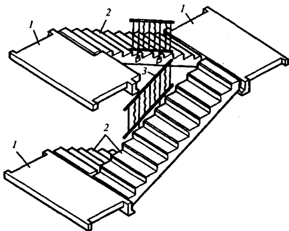
Рис. 3.59. Лестница из крупнооборных элементов: 1 — лестничные площадки; 2 — лестничные марши; 3 — фрагмент ограждения
