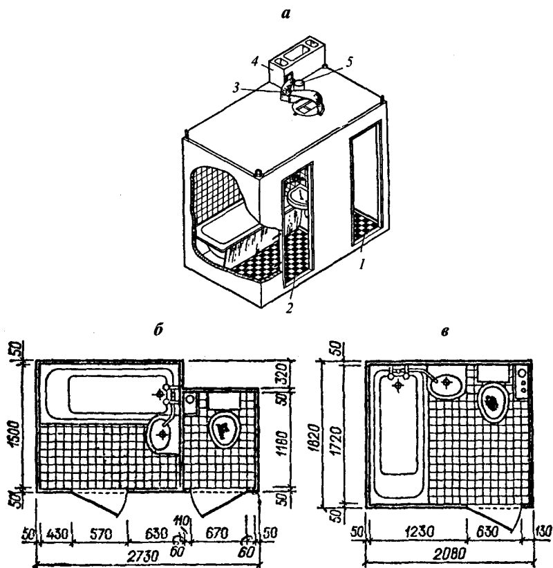
Рис. 4.15. Санитарно-технические кабины:
