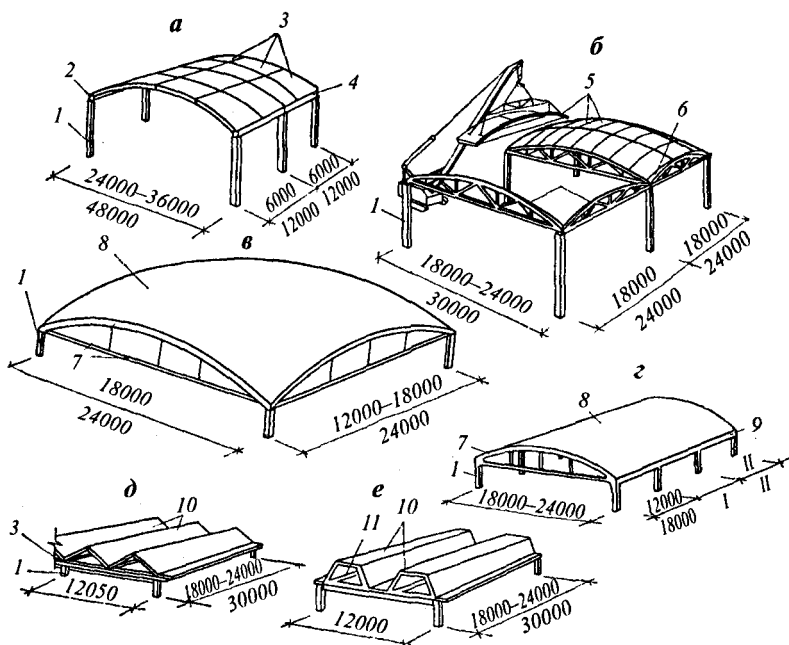
Рис. 6.42. Пространственные покрытия:
