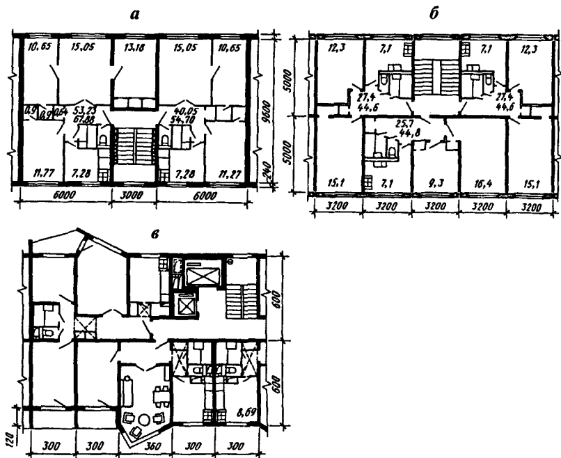
Рис. 2.1. Секции жилых домов: а — двухквартирная 5-этажного дома; б — трехквартирная; в — четырехквартирная 16-этажного дома
