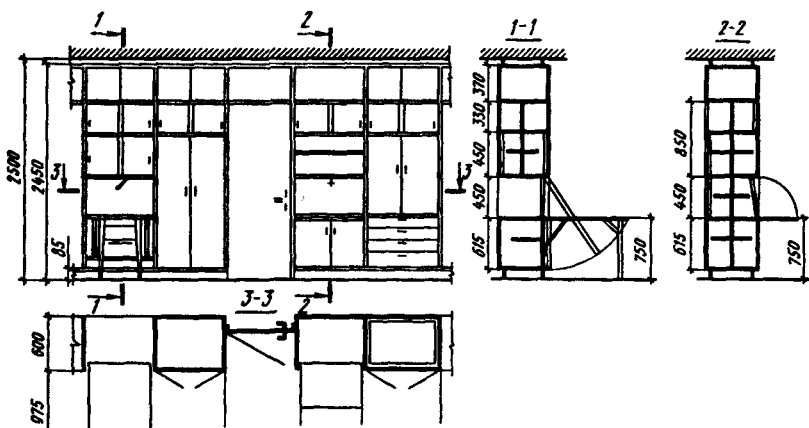
Рис. 3.41. Деревянная перегородка-шкаф
