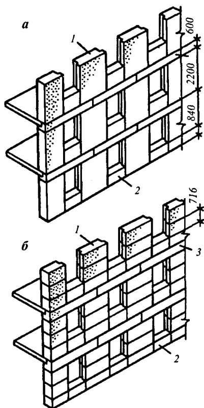
Рис. 4.10. Схемы разрезки стен крупноблочных зданий: а — двухрядная; б — четырехрядная; 1 — простеночный блок; 2 — подоконный блок; 3 — блок-перемычка
