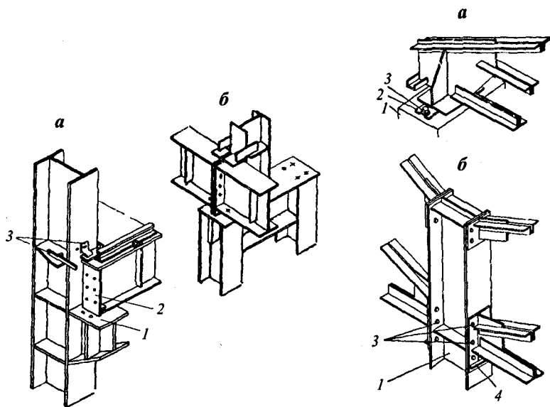
Рис. 6.28. Крепление подкрановых балок: а — к крайней колонне; б — к средней колонне;
