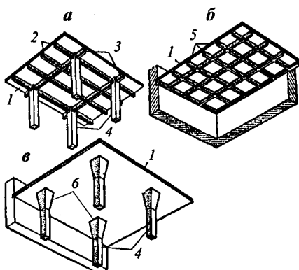
Рис. 3.30. Монолитные железобетонные перекрытия:
