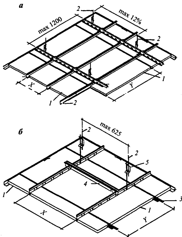
Рис. 3.67. Варианты укладки отделочных потолочных элементов: несъемный (а) и съемный (б) варианты; 1 — потолочная панель; 2 — подвеска; 3 — несущий стальной профиль; 4 — связующий элемент; 5 — регулирующее устройство; X, Y — модульные размеры потолочных элементов
