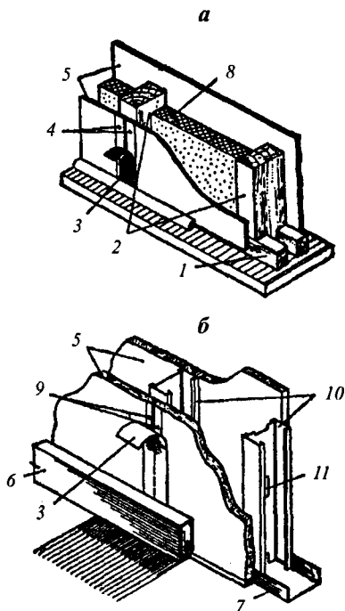
Рис. 3.39. Обшивные перегородки:
