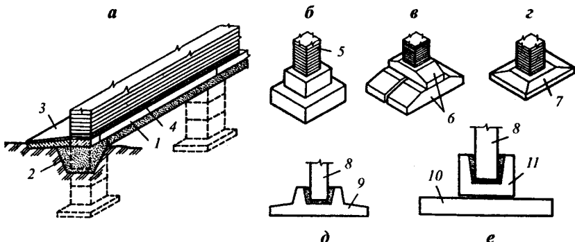
Рис. 3.9. Столбчатые фундаменты:
