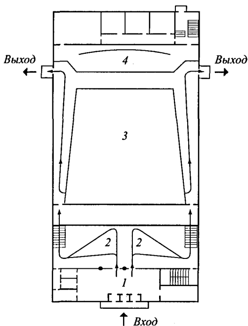
Рис. 2.4. Зальная схема планировки: 1 — вестибюль; 2 — фойе; 3 — зрительный зал; 4 — эстрада
