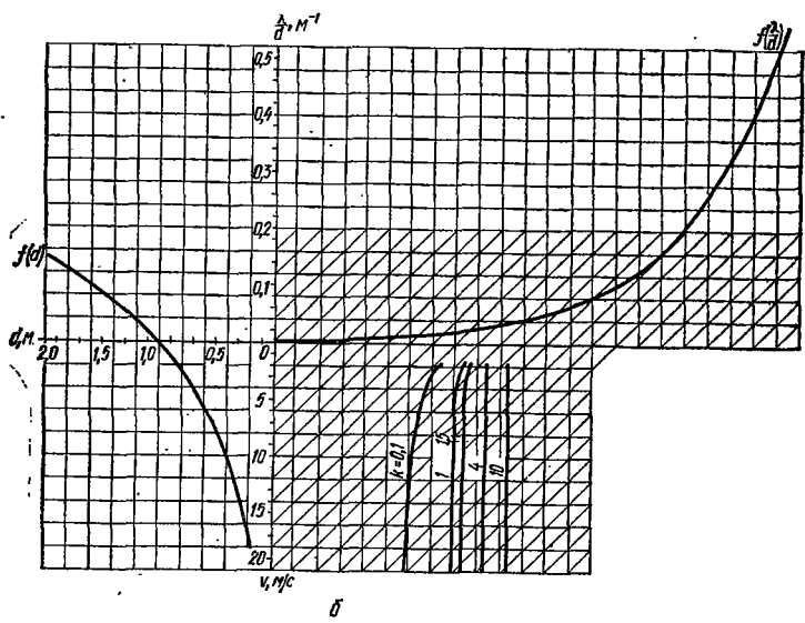
Рис. 4.72. Номограммы для определения величины \lambda/d при скорости воздуха a — до 2 м/с; б — до 20 м/с.
