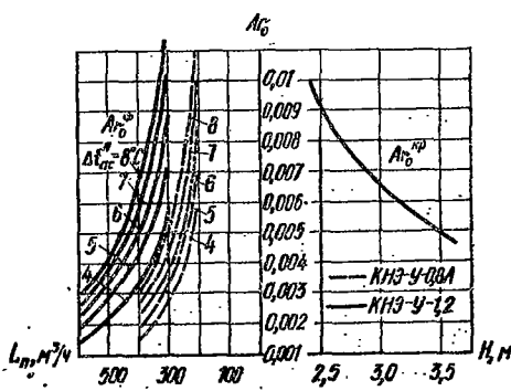
Рис. 4.12. Номограмма для определения критериев Архимеда Ar_0 и Ar_0^{кр} .
