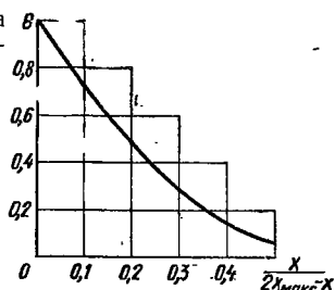
Рис. 4.66. Номограмма для определения величины \Theta .
