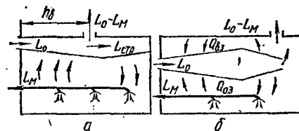
Рис. 4.58. Схемы подачи воздуха ВР, расположенными выше рабочей зоны, когда параметры его в рабочей зоне формируются обратными потоками: а — настилаящаяся струя; б — ненастилаящаяся струя.
