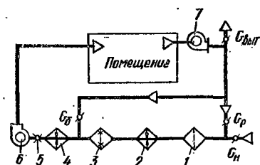
Рис. 4.8. Структурная схема СКВ с первой и второй рециркуляциями:
