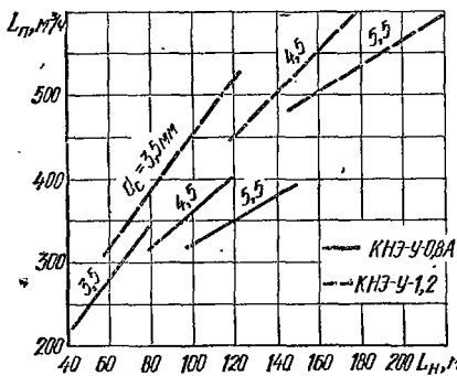
Рис. 4.11. Номограмма для подбора сопел ЭКД.
