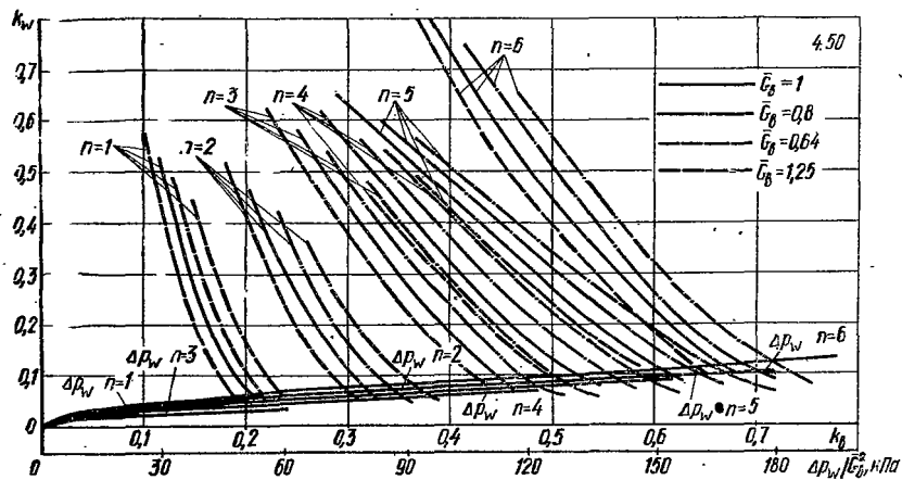
Рис. 4.49—4.54. Номограммы для расчета воздухонагревателей и воздухоохлаждателей кондиционеров Кд (номер рисунка указан в правом верхнем углу номограммы).
