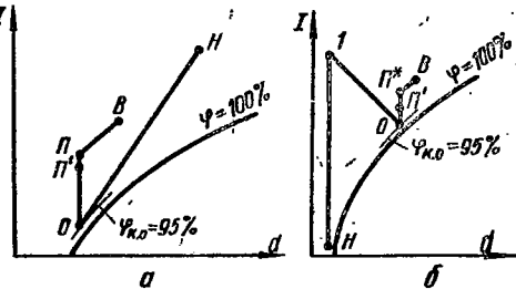
Рис. 4.5. Процессы обработки наружного воздуха в проточной СКВ в летний (а) и зимний (б) периоды.
