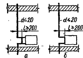
Рис. 3.3. Монтажные положения неизолированных трубопроводов систем отопления:
