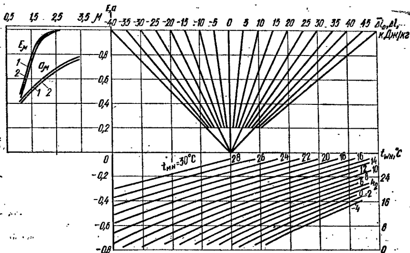
Рис. 4.19. Номограмма для расчета камер орошения ОКС (перекрестноточная схема):
