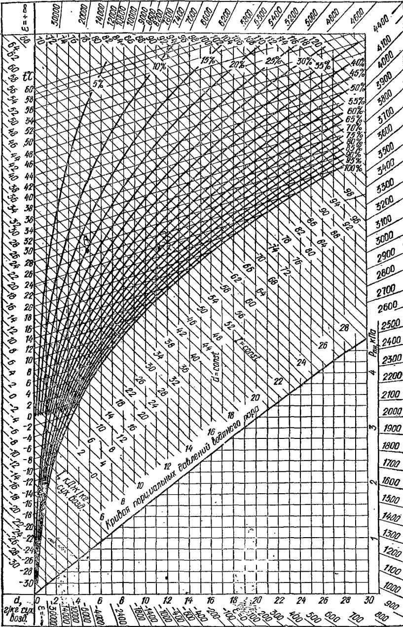
Рис. 4.3. I — d-диаграмма ( p_6 = 1010 гПа).
