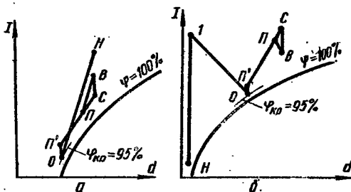
Рис. 4.15. Процессы обработки воздуха в летний (а) и зимний (б) периоды (к примеру расчета).
