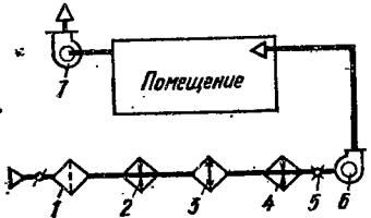
Рис. 4.4. Структурная схема проточной СКВ:
