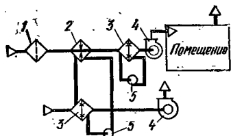
Рис. 4.16. Структурная схема СКВ с двухступенчатым испарительным охлаждением воздуха:
