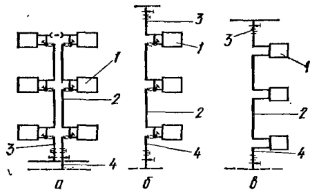
Рис. 3.9. Элементы одитрубного стояка:
