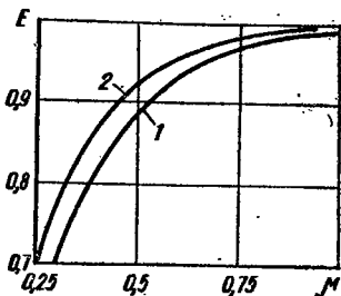
Рис. 4.18. Номограмма для расчета камер орошения ОКС (противоточная схема):
