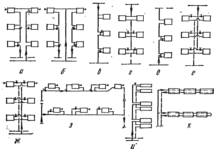
Рис. 3.1. Принципиальные схемы стояков систем водяного отопления: а, б — П- и Т-образные стояки вертикальной одноконтурной системы с нижней разводкой; в, г — стояки вертикальной одноконтурной системы с верхней разводкой с односторонним и двусторонним присоединением приборов; д — стояк вертикальной одноконтурной системы с опрокинутой циркуляцией; е, ж — стояки двухконтурной системы с верхней и нижней разводкой; з — стояк горизонтальной одноконтурной системы; и, к — стояки вертикальной и горизонтальной бифилярной системы.
