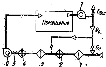
Рис. 4.6. Структурная схема СКВ с первой рециркуляцией:
