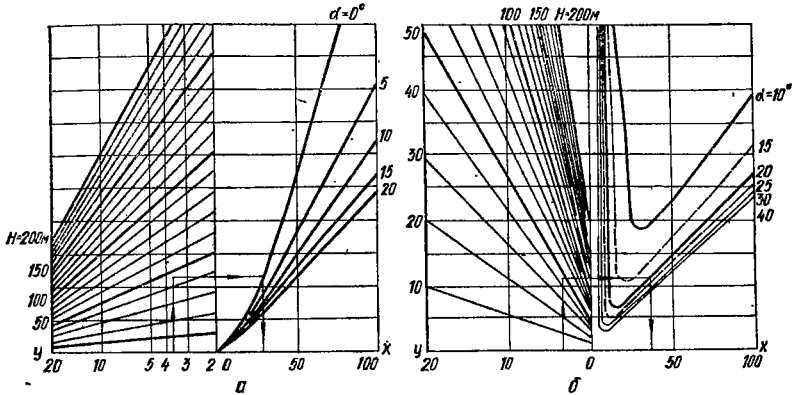
Рис. 4.64. Номограмма для определения горизонтального расстояния от ВР до входа геометрической оси струи в обслуживаемую зону при подаче воздуха под углом к горизонтальной плоскости: а — охлажденный воздух; б — нагретый воздух.
