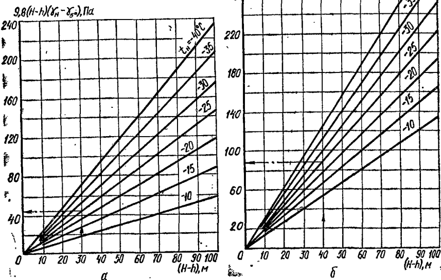
Рис. 2.3. Номограммы для определения величин 9,8(H-h)(\gamma_H - \gamma_{5^0}) (а) и 9,8(H-h)(\gamma_H - \gamma_{18^0}) (б).
