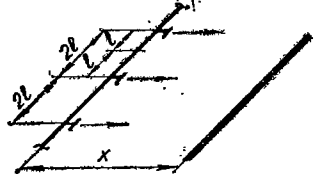
Рис. 4.69. Схема установок воздушораспределителей в ряд.
