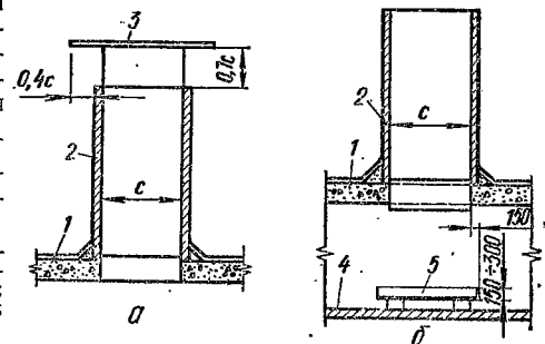
Рис. 4.2. Схема устройства вытяжной шахты из теплого чердака:
