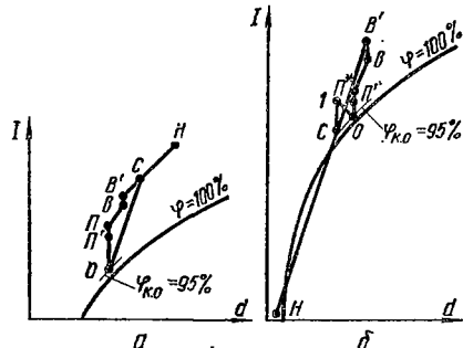
Рис. 4.7. Процессы обработки воздуха в летний (а) и зимний (б) периоды в СКВ с первой рециркуляцией.
