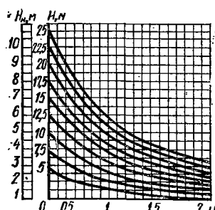
Рис. 3.7. Номограмма для определения напора, создаваемого элеватором в системе водяного отопления ( H_n — располагаемый напор для циркуляции в системе после элеватора; H — разность напоров в подающем и обратном трубопроводах тепловой сети на вводе в здания).
