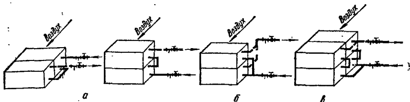
Рис. 4.70. Схемы соединения калориферов по воде:
