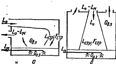
Рис. 4.56. Схемы подачи воздуха ВР, расположенными выше рабочей зоны, при удалении его вие зоны непосредственного воздействия струи: а — настилаящаяся струя; б — ненастилаящаяся струя.
