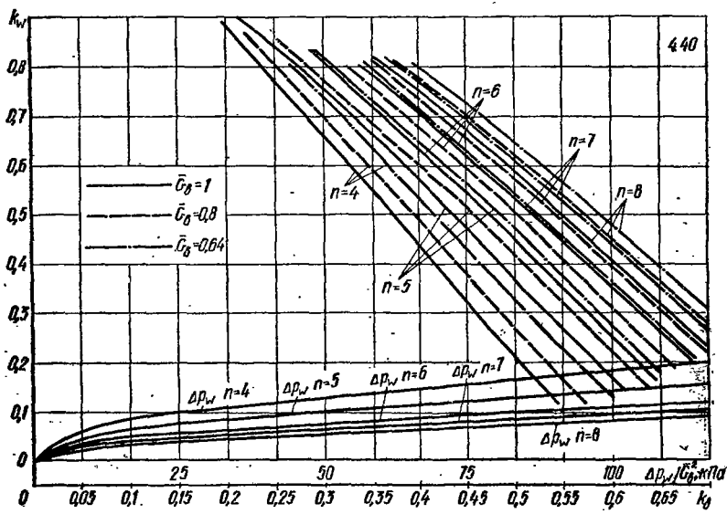
Рис. 4.40—4.47. Номограммы для расчета воздухоохладителей и блоков теплообмена (номер рисунка указан в правом верхнем углу номограммы).
