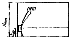
Рис. 4.61. Схема подачи воздуха закрученными струями горизонтально ВР, расположенными в рабочей зоне.
