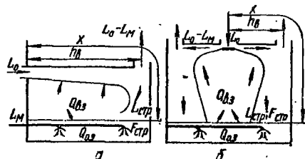
Рис. 4.57. Схемы подачи воздуха ВР, расположенными выше рабочей зоны, при удалении его в зоне непосредственного воздействия струи: а — плоская, или компактная струя; б — вверная струя.
